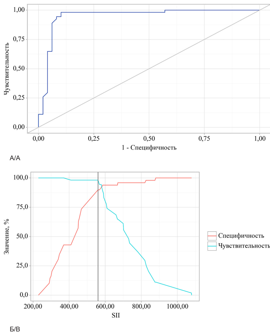
Рис. 2. ROC-кривая, характеризующая дискриминационную способность SII при прогнозировании «non-dipper» (А), анализ чувствительности и специфичности модели в зависимости от пороговых значений (Б).
